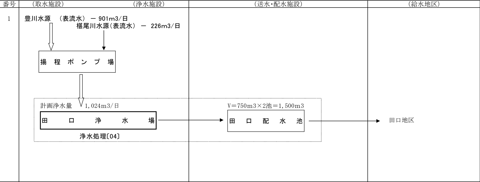
(令和6年度) 設楽町簡易水道(田口)給水フロー図
