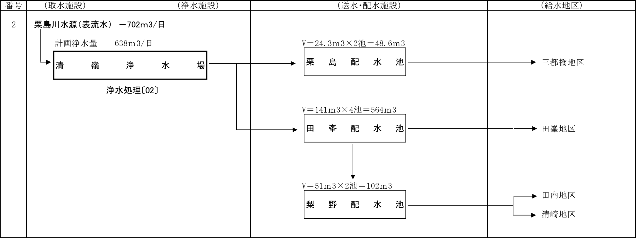
(令和6年度) 設楽町簡易水道(清嶺)給水フロー図
