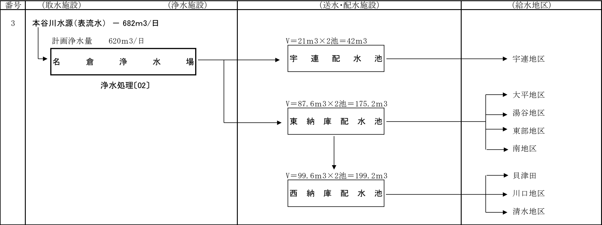
(令和6年度) 設楽町簡易水道(名倉)給水フロー図
