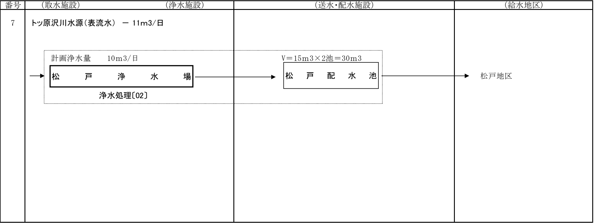
(令和6年度) 設楽町簡易水道(松戸) 給水フロー図
