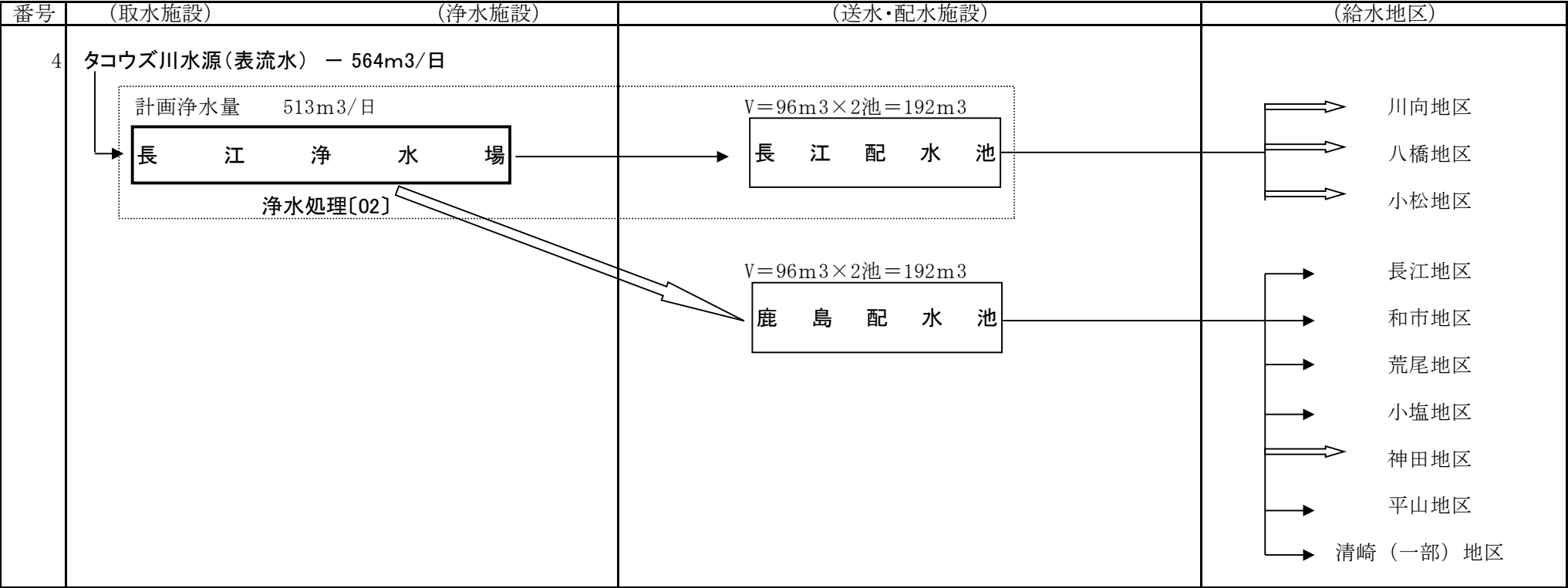
(令和6年度) 設楽町簡易水道(田口第2地区) 給水フロー図
