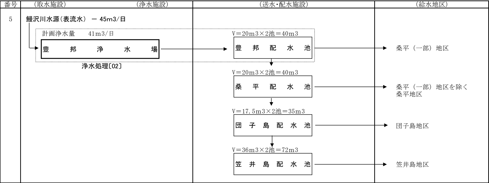
(令和6年度) 設楽町簡易水道(豊邦) 給水フロー図
